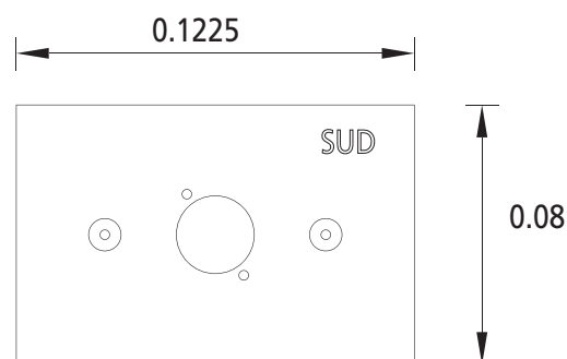
Modelo XLR simple
